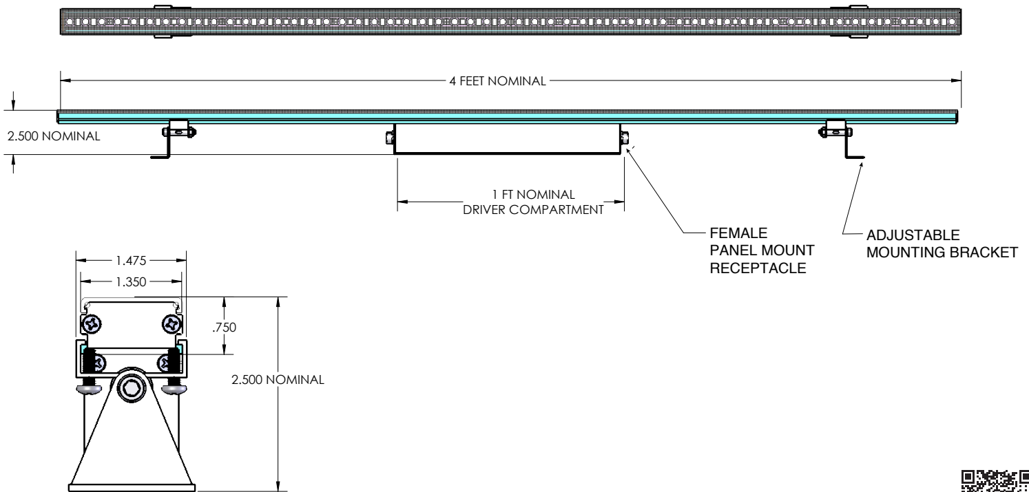
SCALE 1:1
